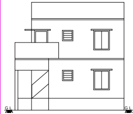
ELEVATION
