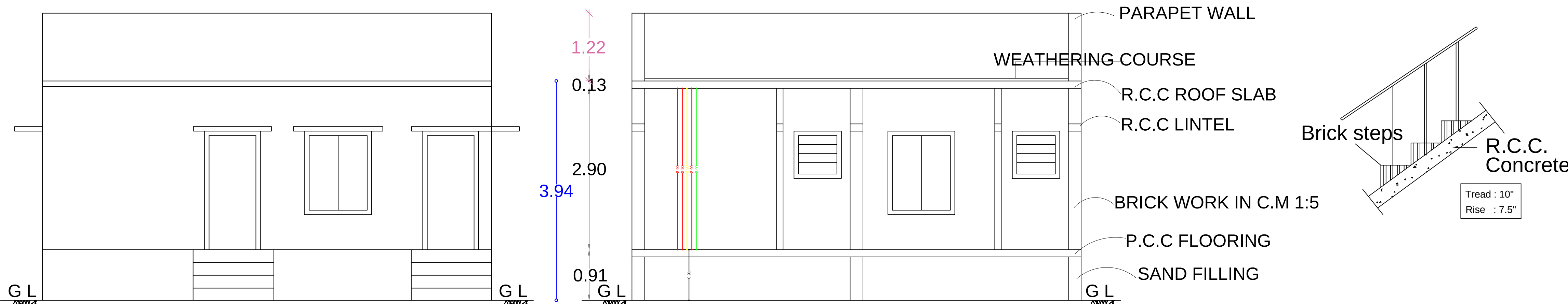
ELEVATION
