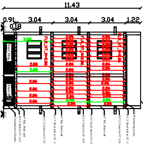
SECTION 'RK'
