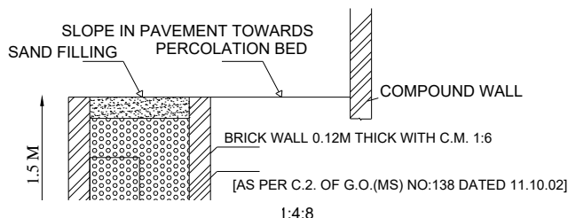
PER PERCOLATION BED
