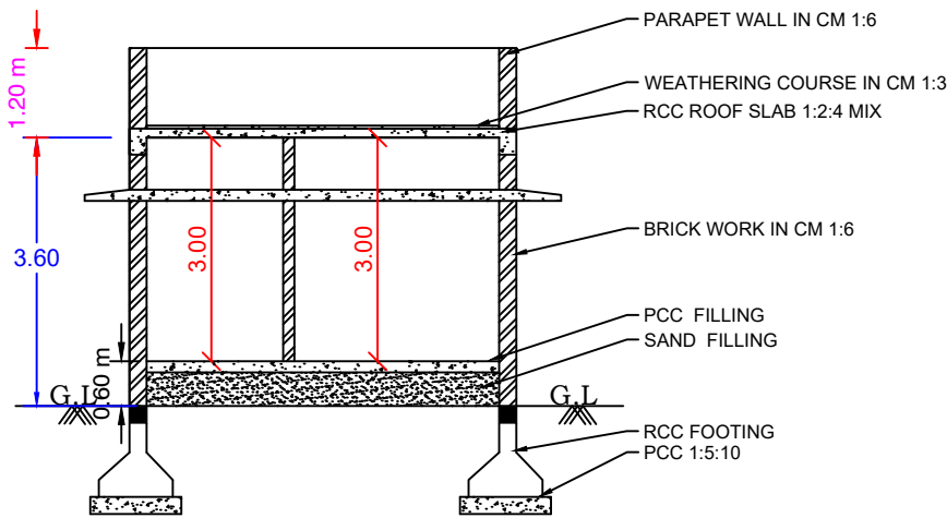
SECTION - AB
