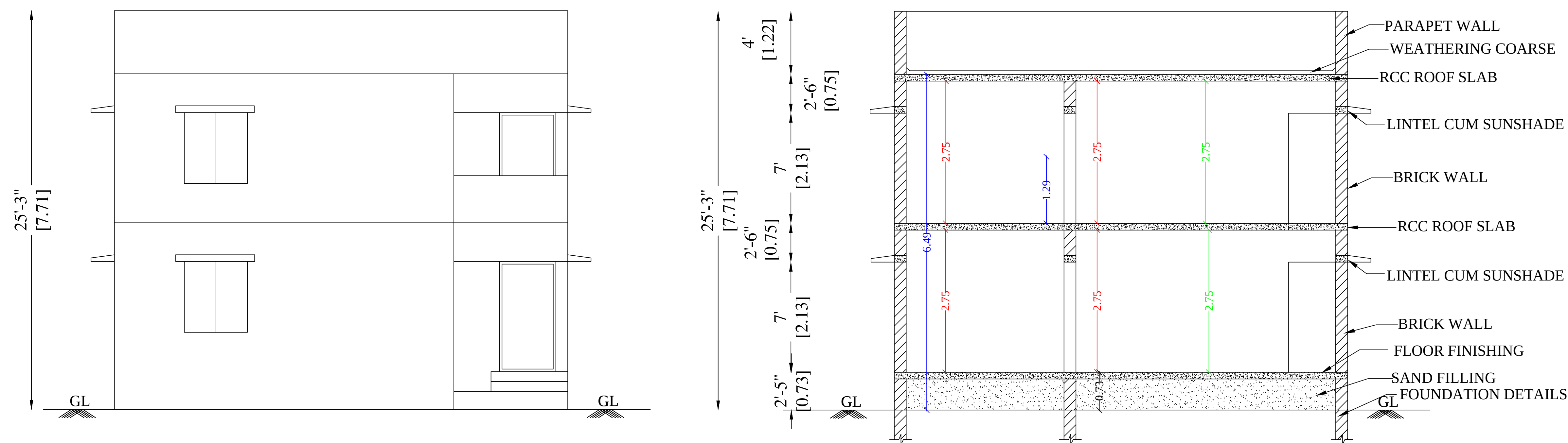
ELEVATION
