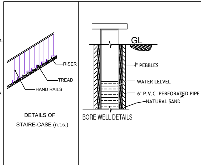
DETAILS OF STAIRCASE (n.l.s.)
