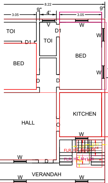
F.F. PLAN
