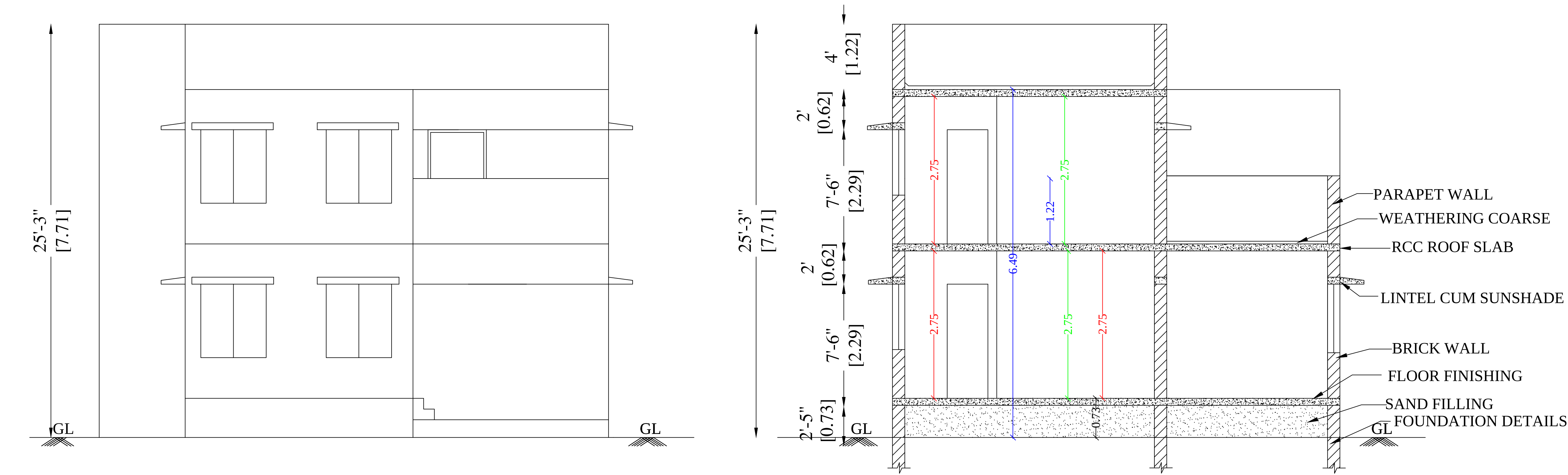
ELEVATION
