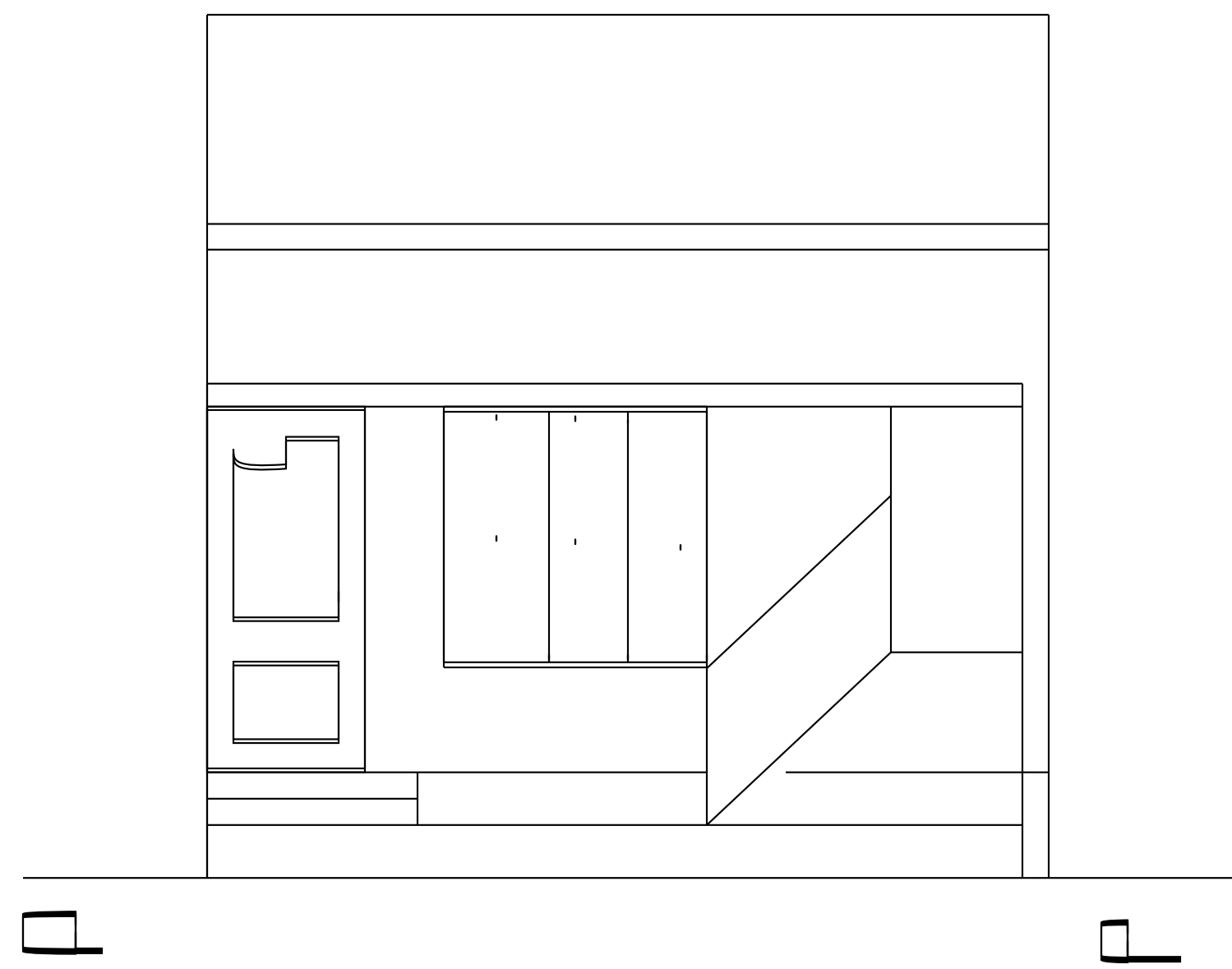
SECTION A-A
