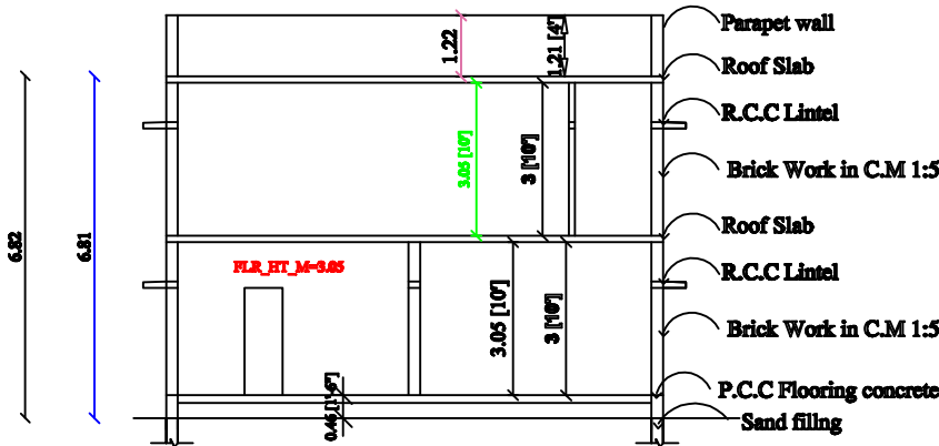
SECTIO ON"AA"
