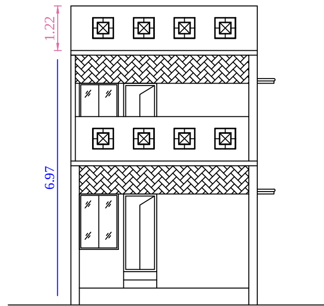
ELEVATION
