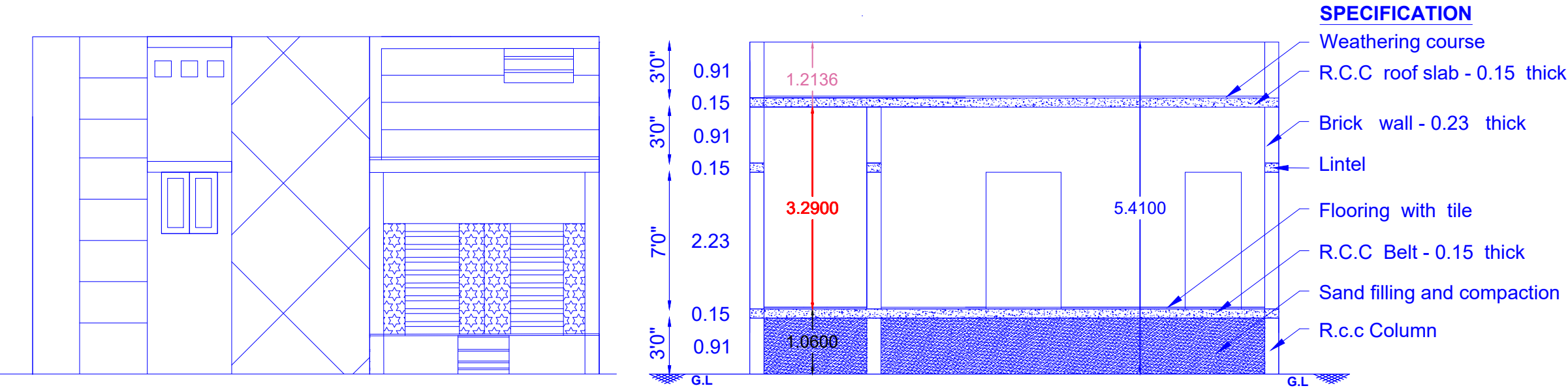
ELEVATION
