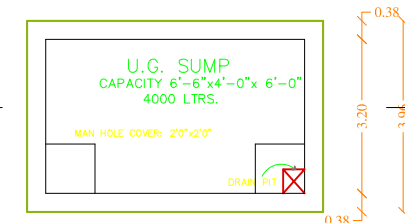
U.G. SUMP
