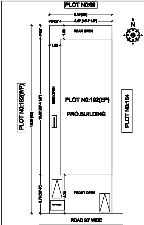
SITE-PLAN
