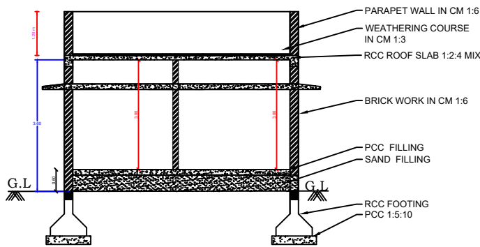
SECTION - AB
