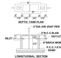
LONGITUDINAL SECTION
