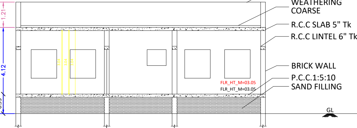
SECTION -AB
