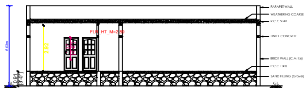
ELEVATION
