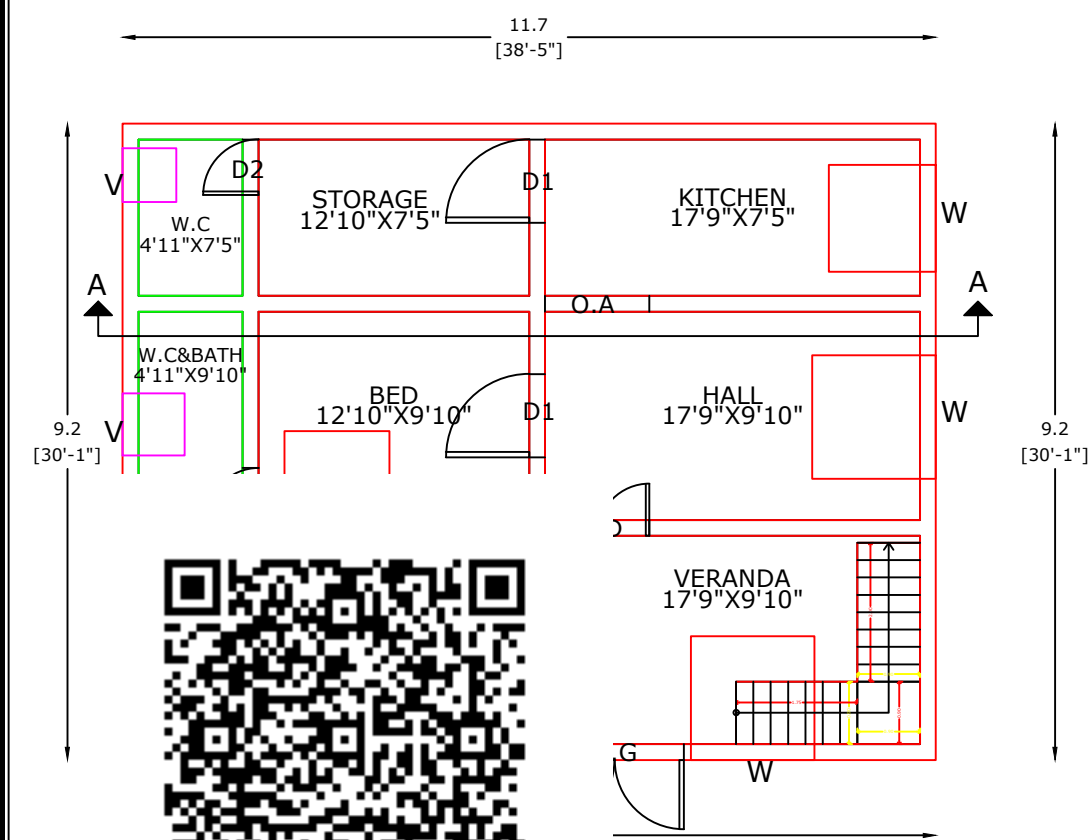
DOOR PLAN
