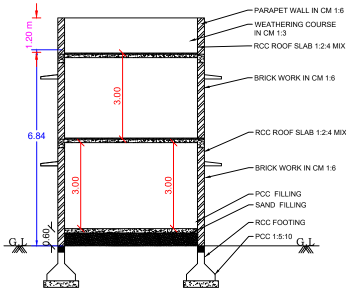
SECTION - AB
