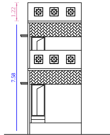
ELEVATION
