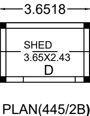
PLAN(445/2B)
