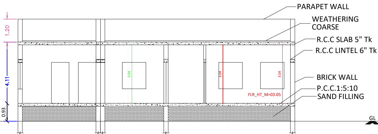
SECTION -AB
