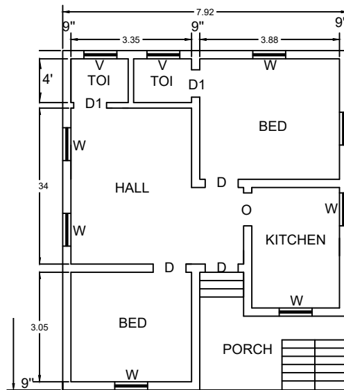
F.F. PLAN
