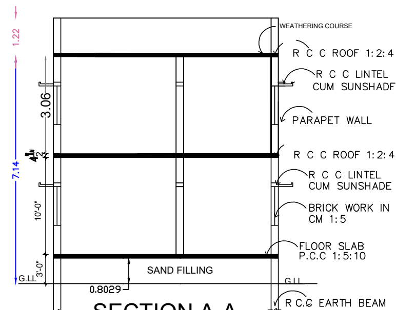
SECTION A-A
