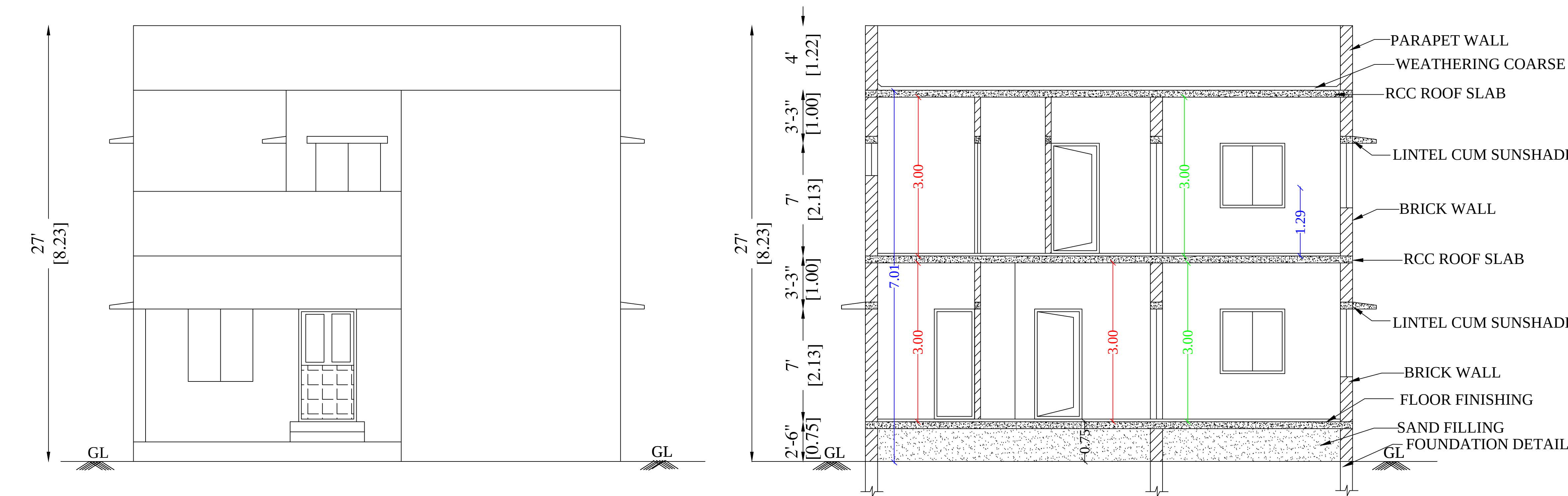
ELEVATION
