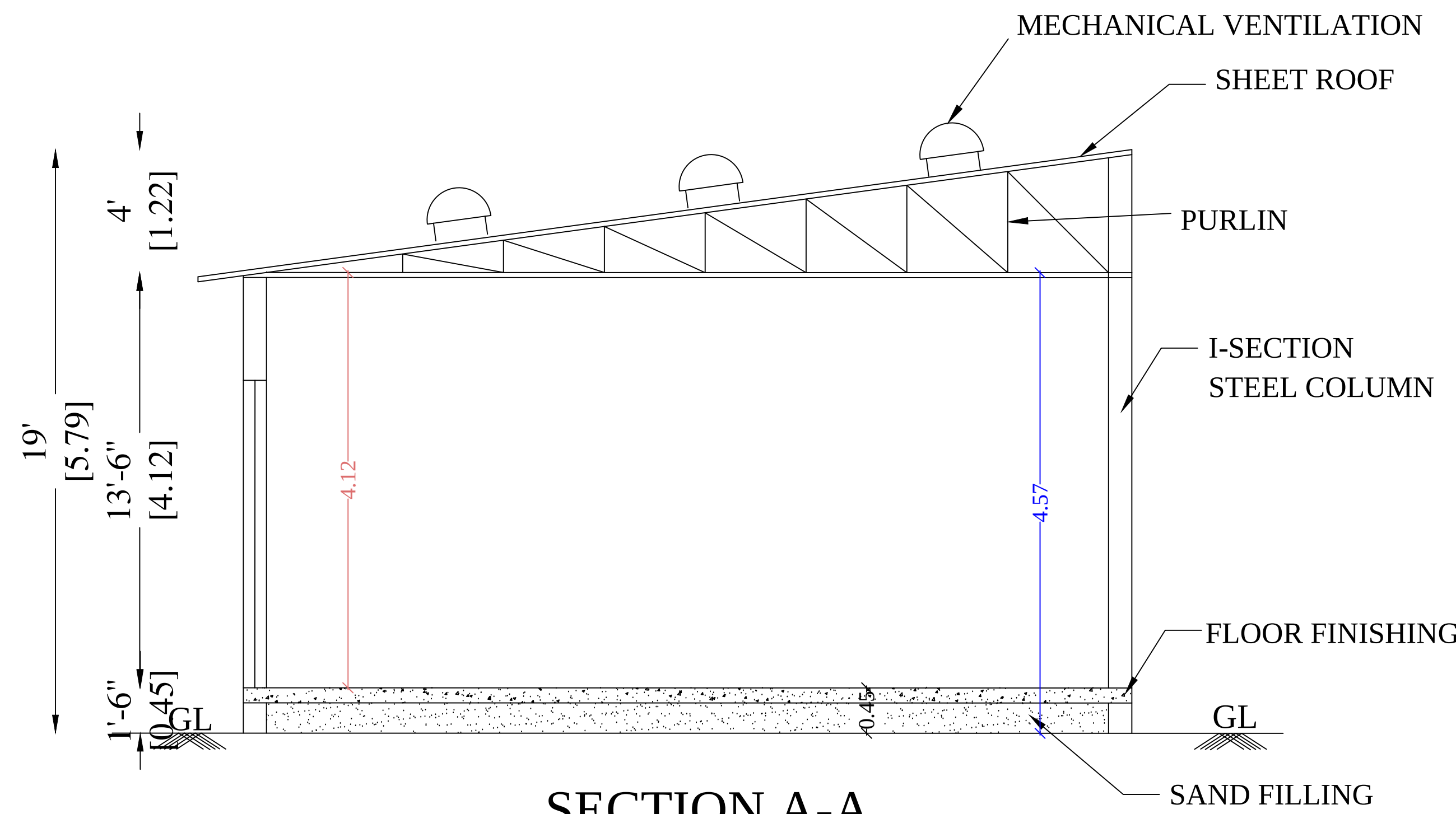
SECTION A-A
