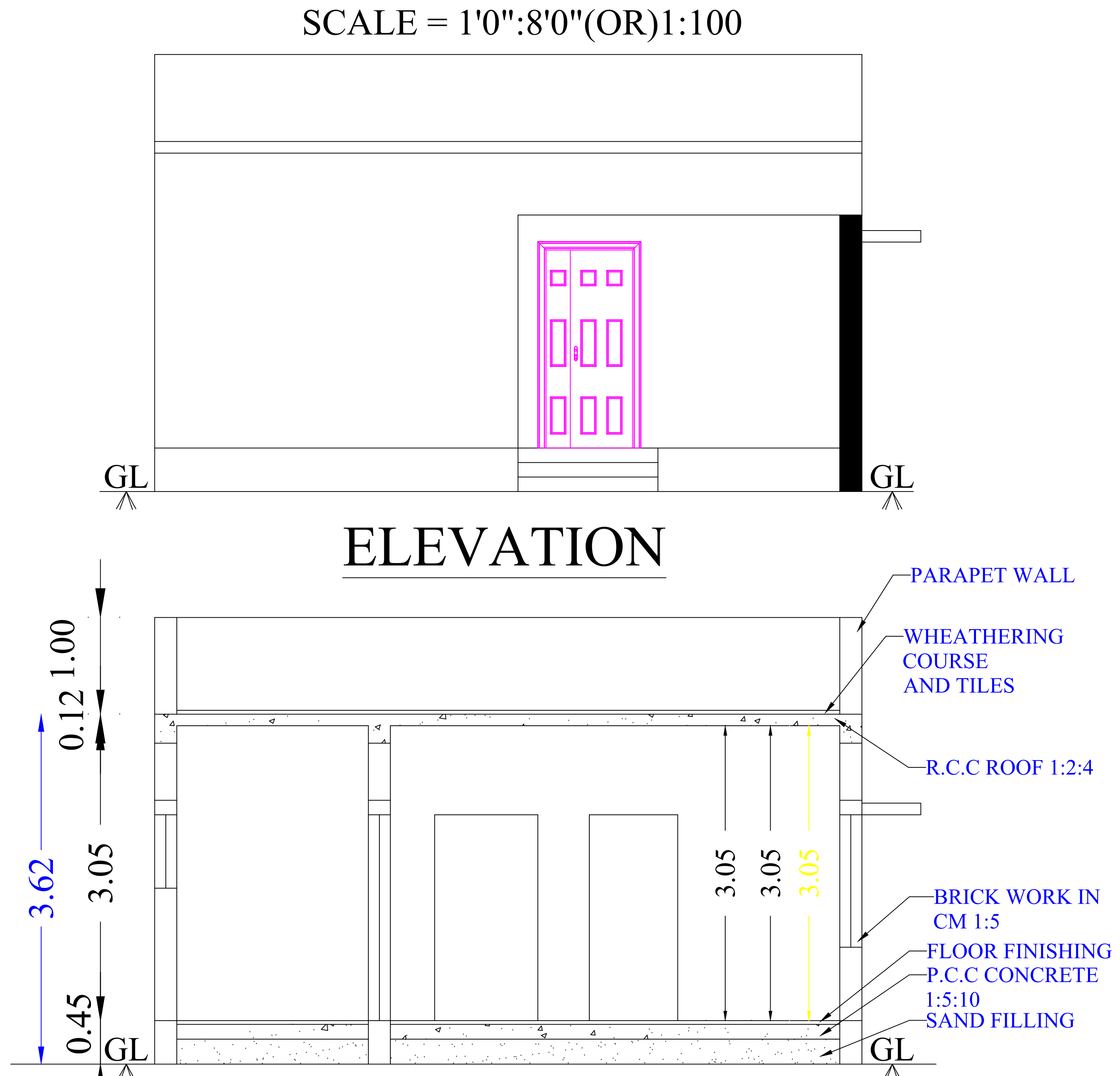
SECTION A-A
