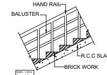
DETAILS OF STAIRCASE (N.T.S)
