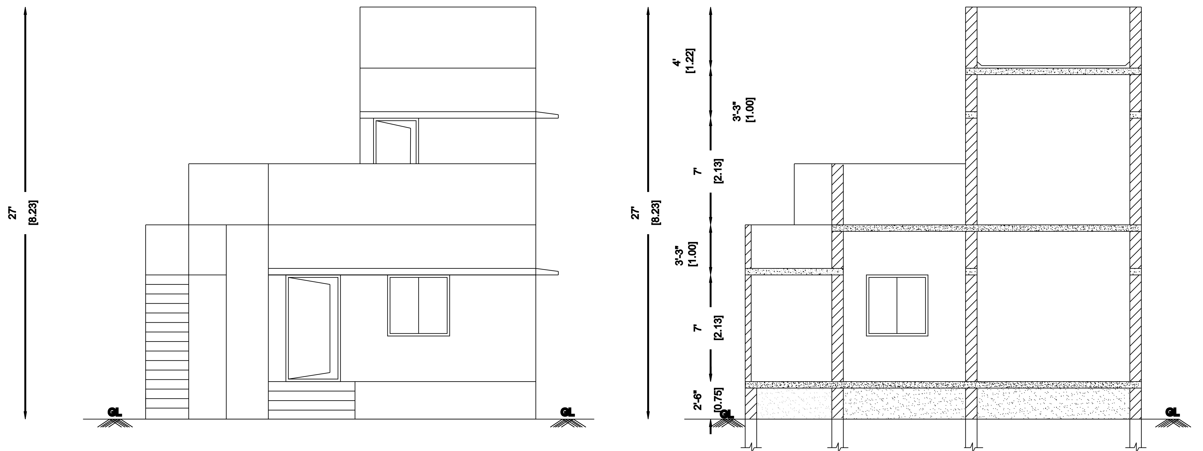
ELEVATION
