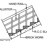
DETAILS OF STAIRCASE (N.T.S.)
