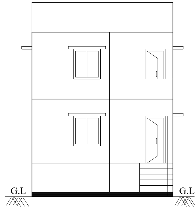
ELEVATION
