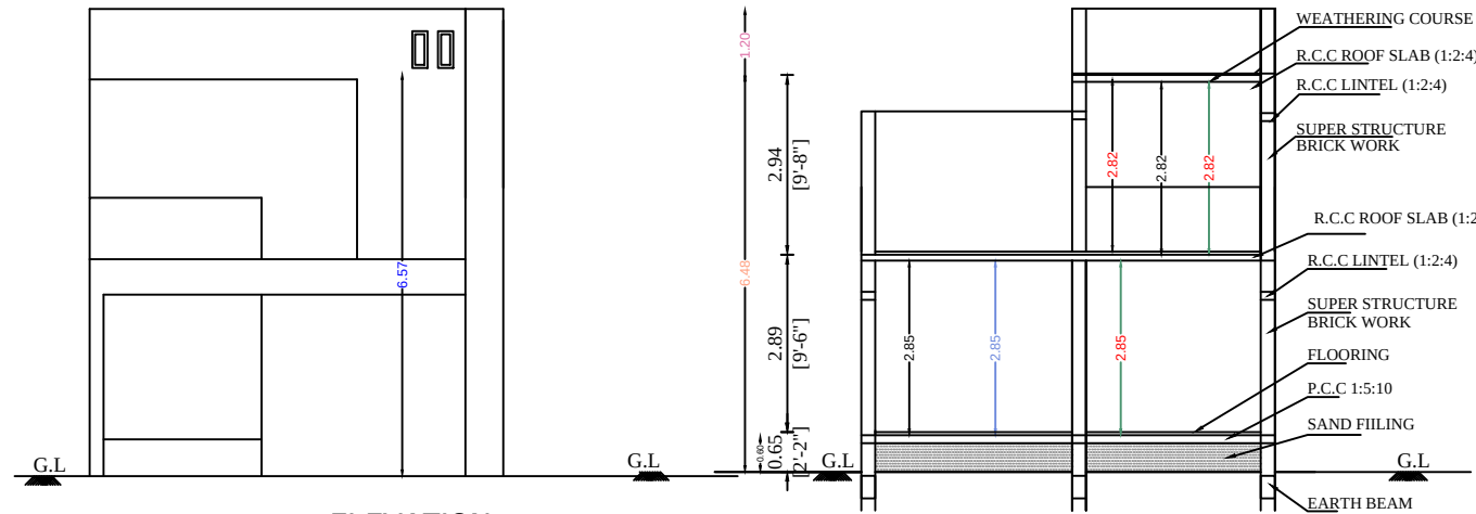
ELEVATION
