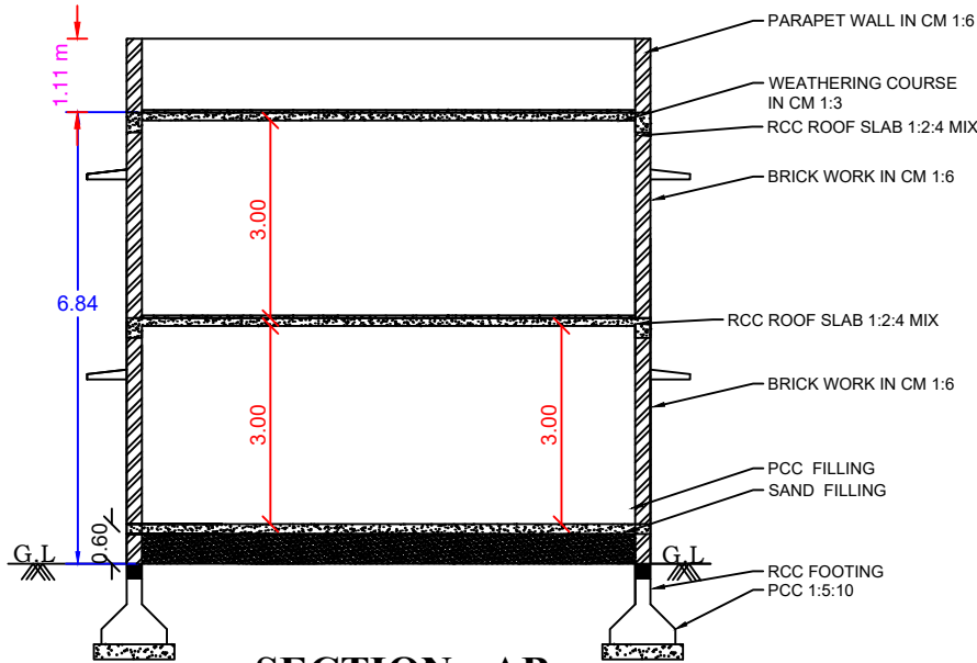
SECTION - AB
