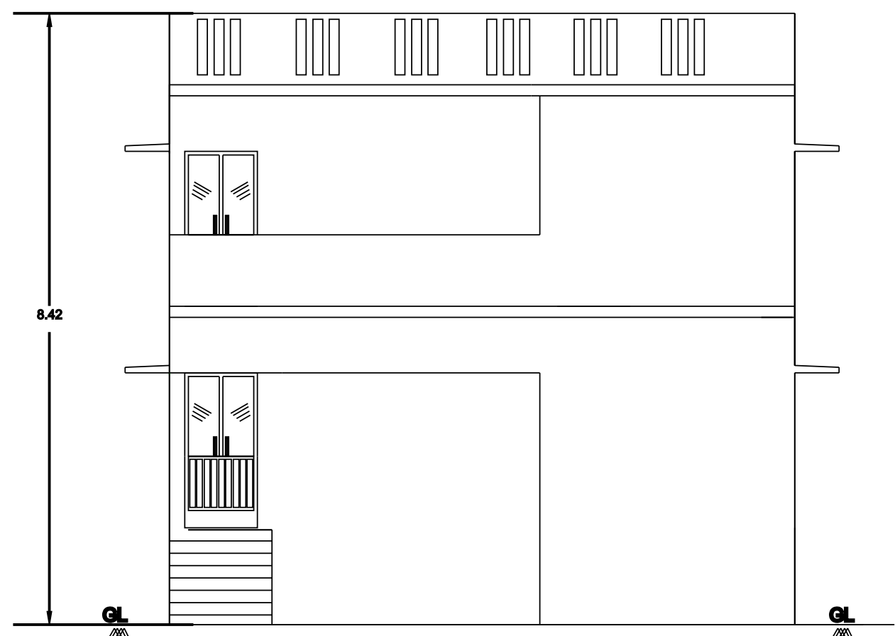
ELEVATION
