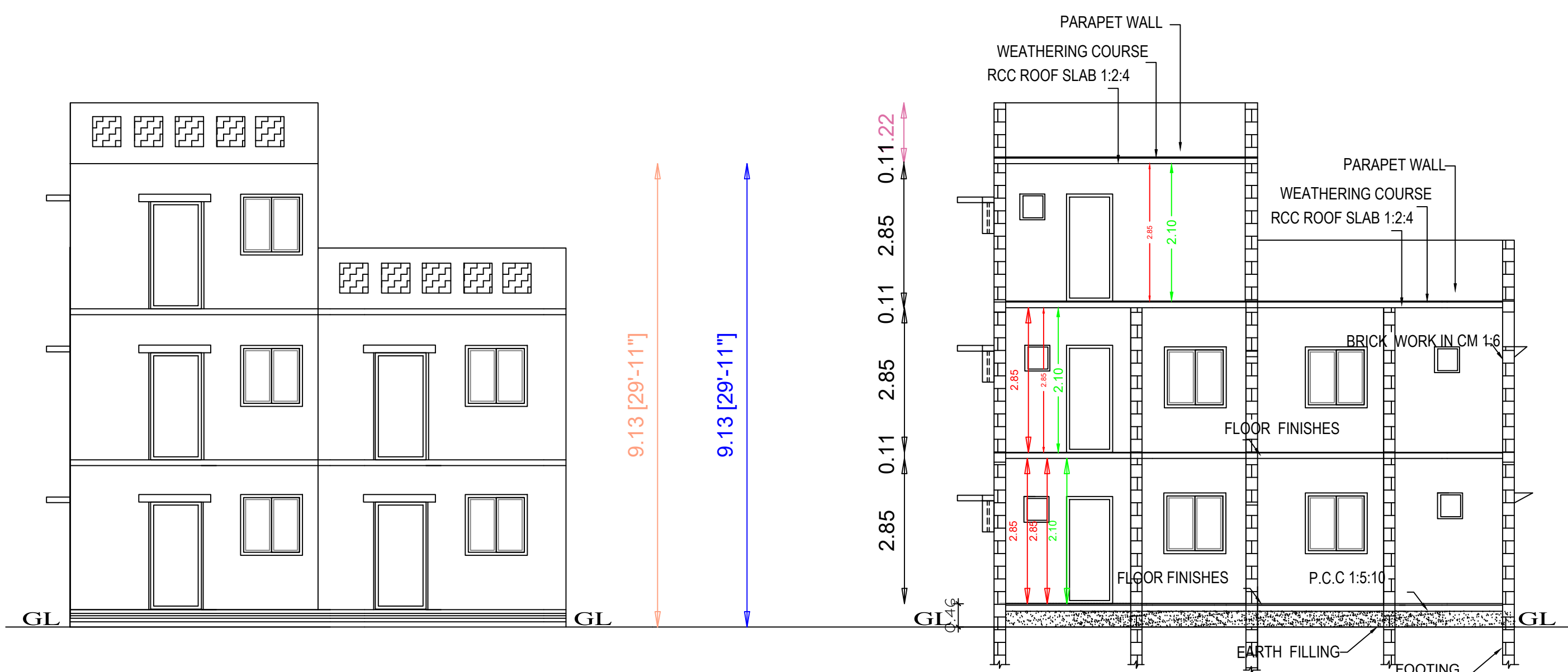
ELEVATION
