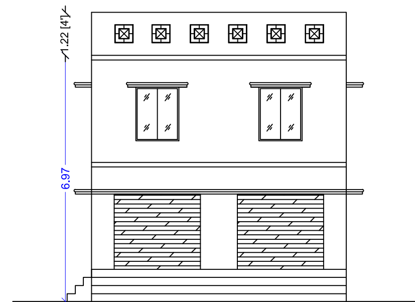
ELEVATION
