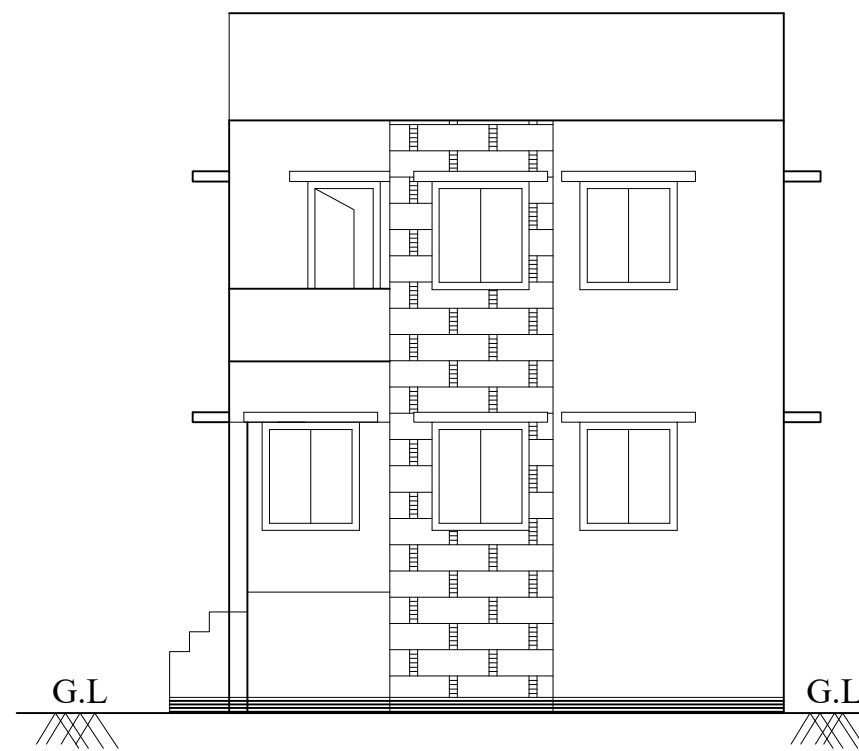
ELEVATION
