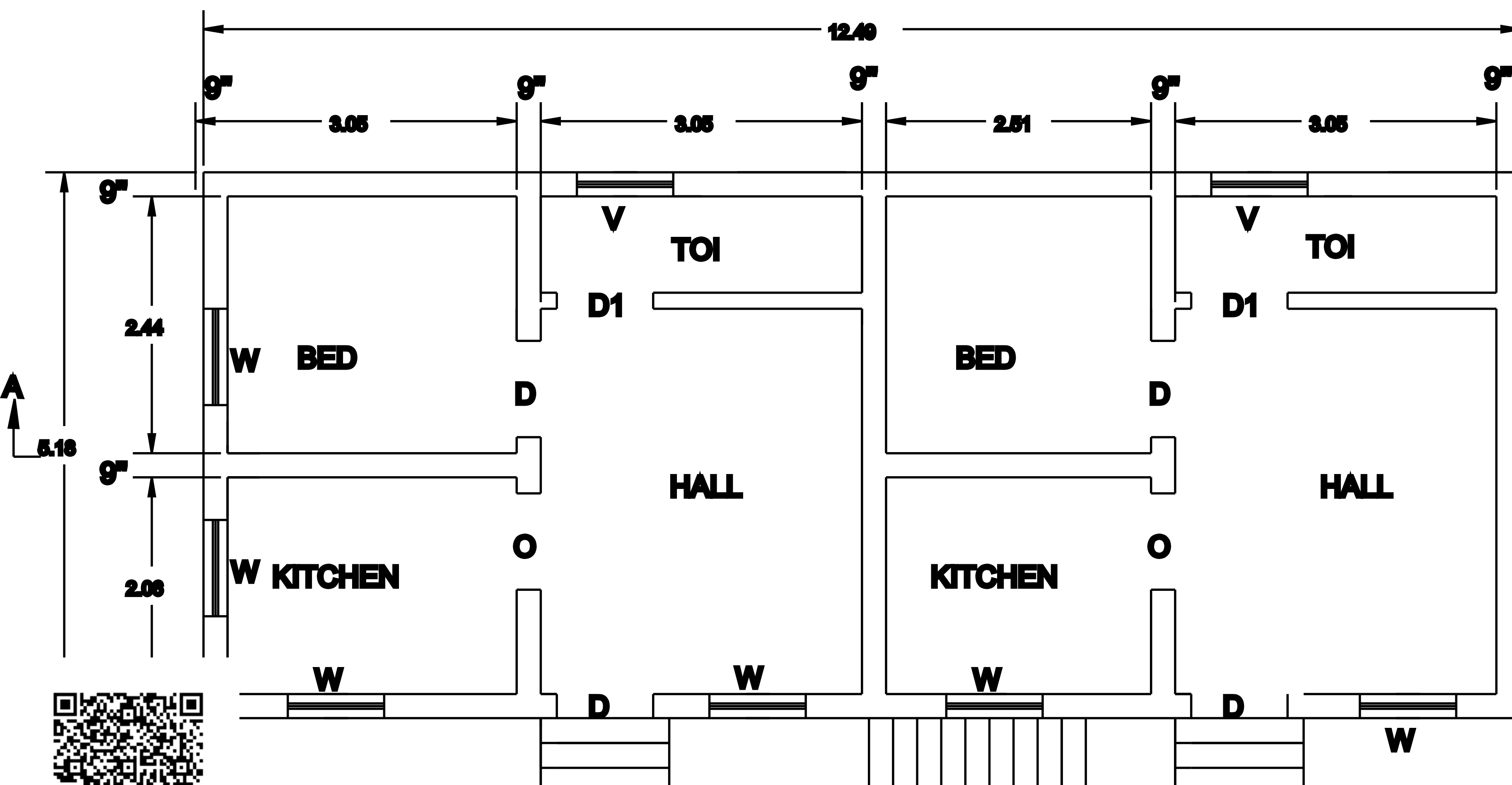
G.F.PLAN
