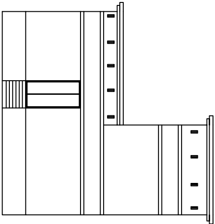
ELEVATION
