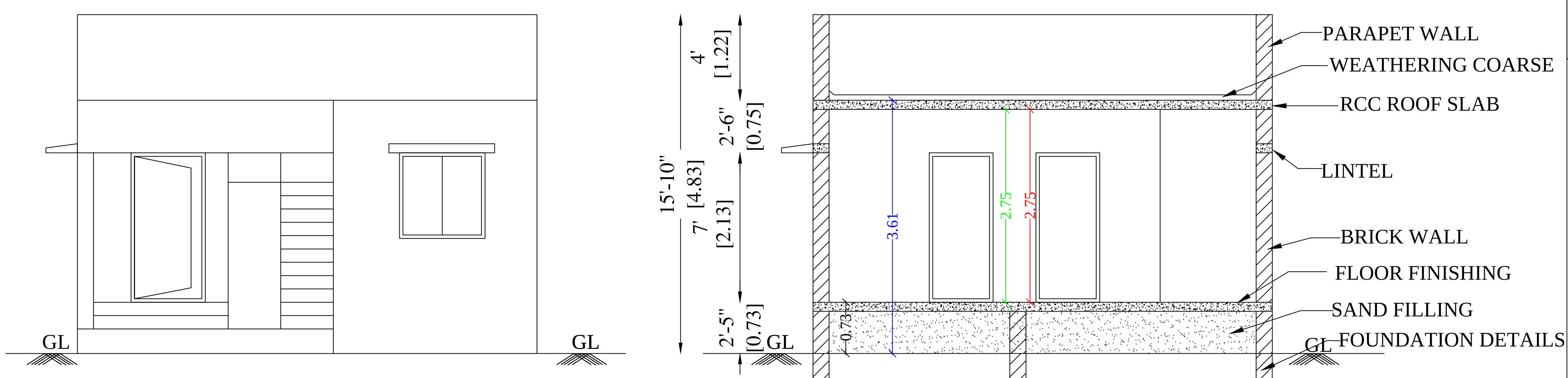
ELEVATION
