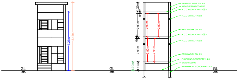
ELEVATION
