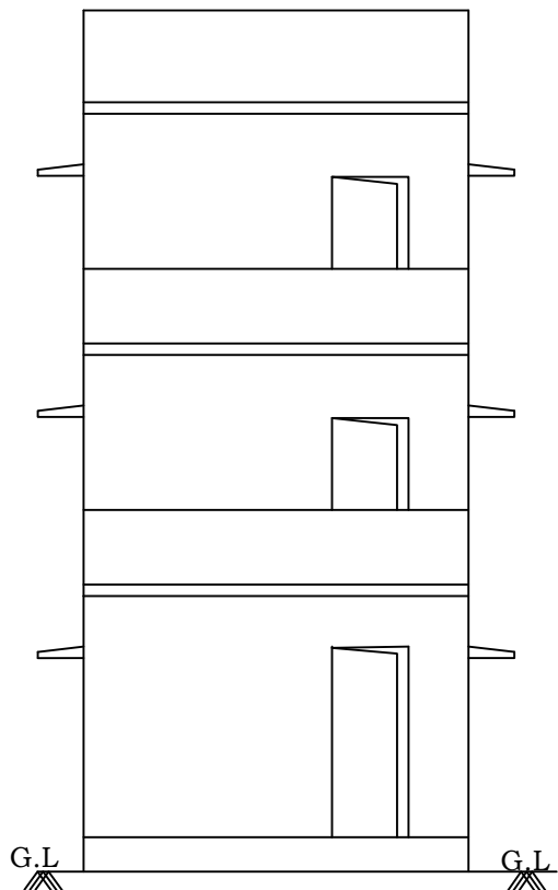
ELEVATION
