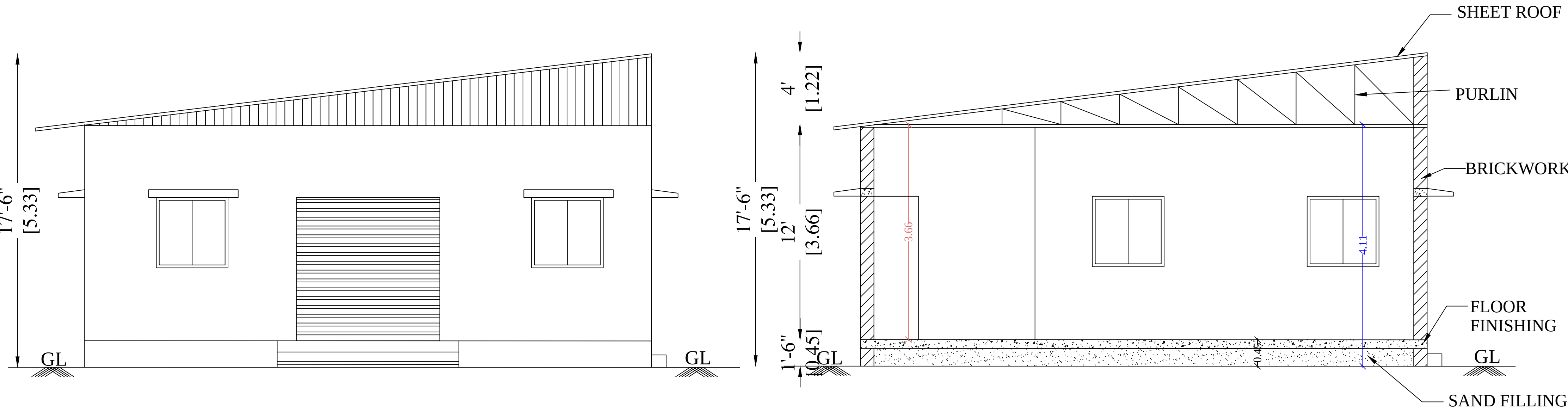
ELEVATION
