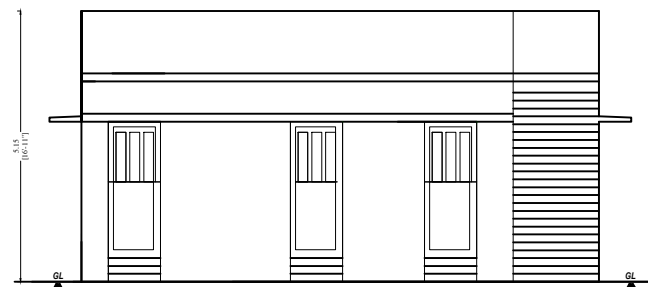
ELEVATION
