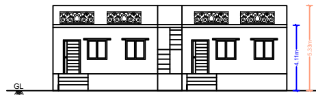
ELEVATION
