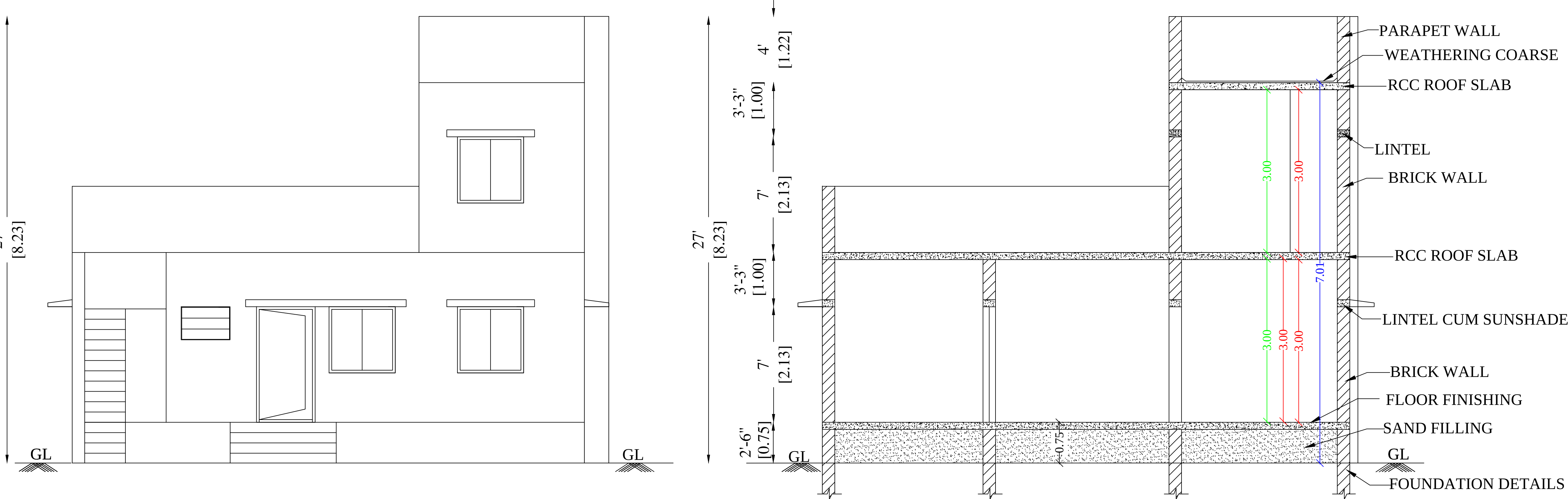
ELEVATION
