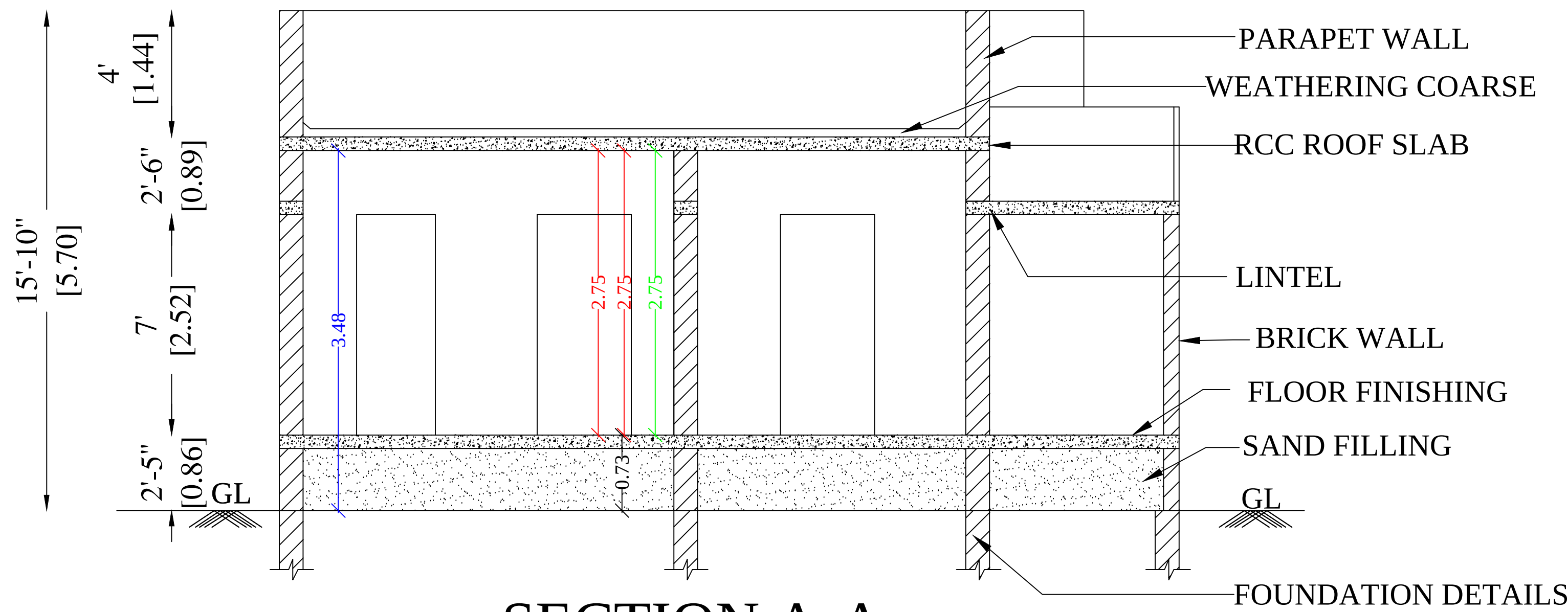
SECTION A-A
