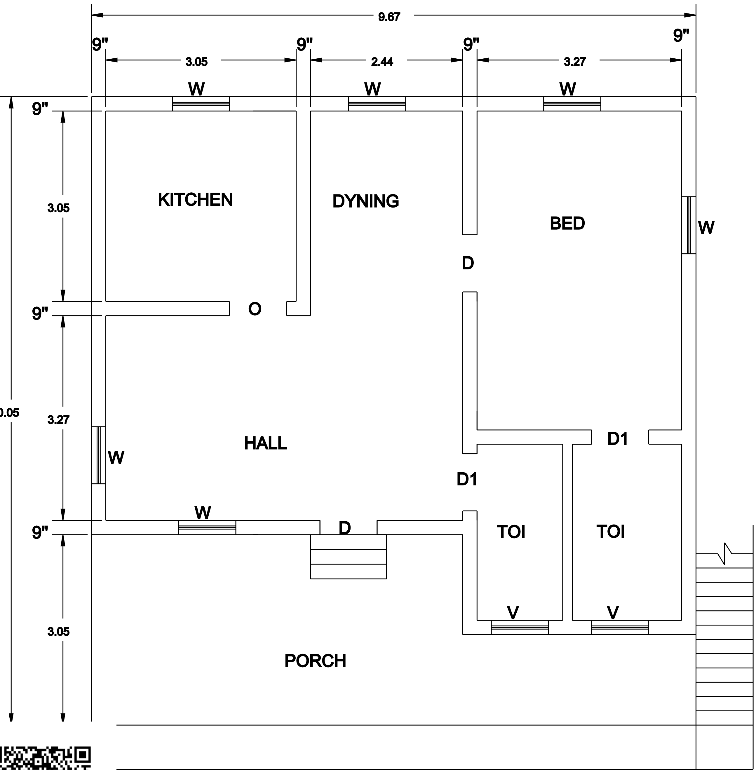
EXISTING G.F PLAN
